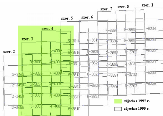
Rys. 2. Fotoszkic dla zdjęć lotniczych z lat 90-tych.
